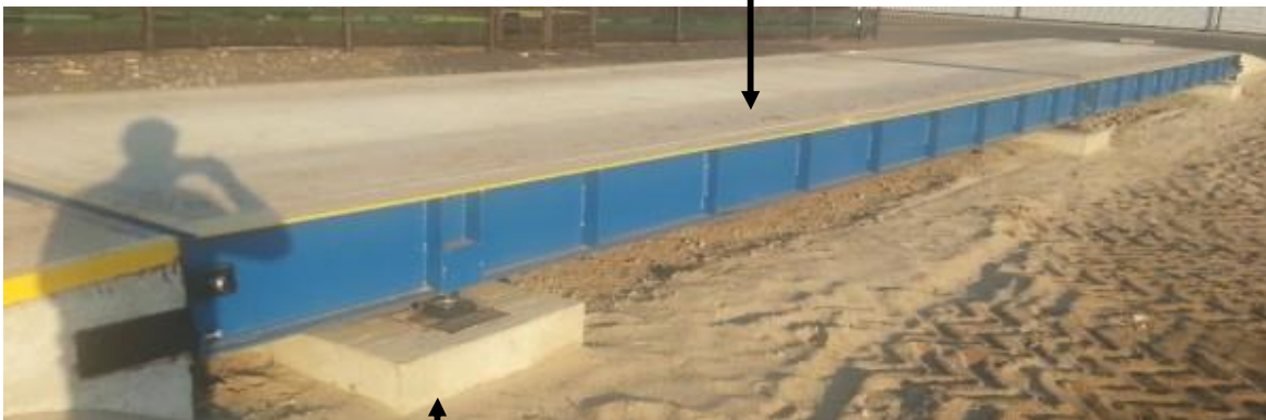
Bauseitige Streifenfundamente / 3 bei 12m - 4 bei 18m Brücke
