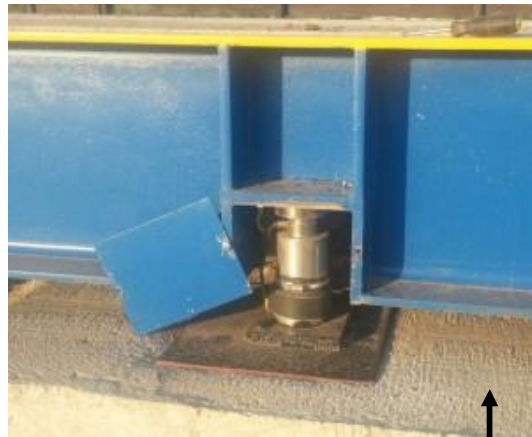
Verbindung der 6m langen Segmente 2 Segmente bei 12m 3 Segmente bei 18m
